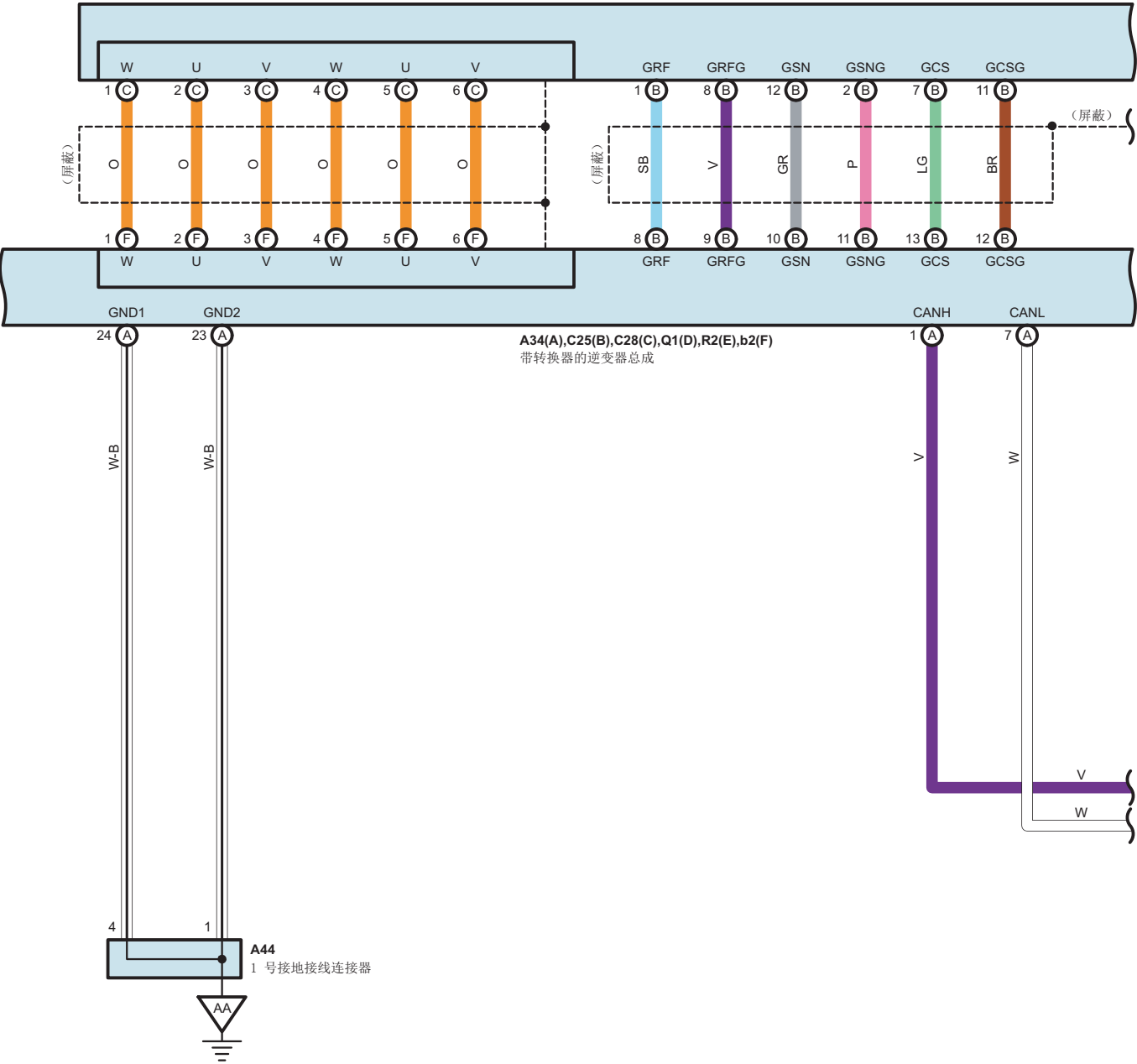
C26(A),C27(B),b1(C) 混合动力车辆传动桥总成
